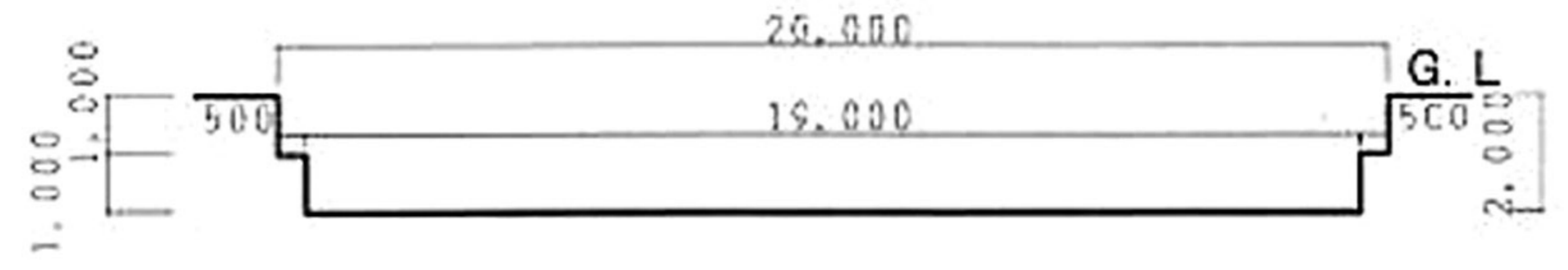
E-E' 断面図
