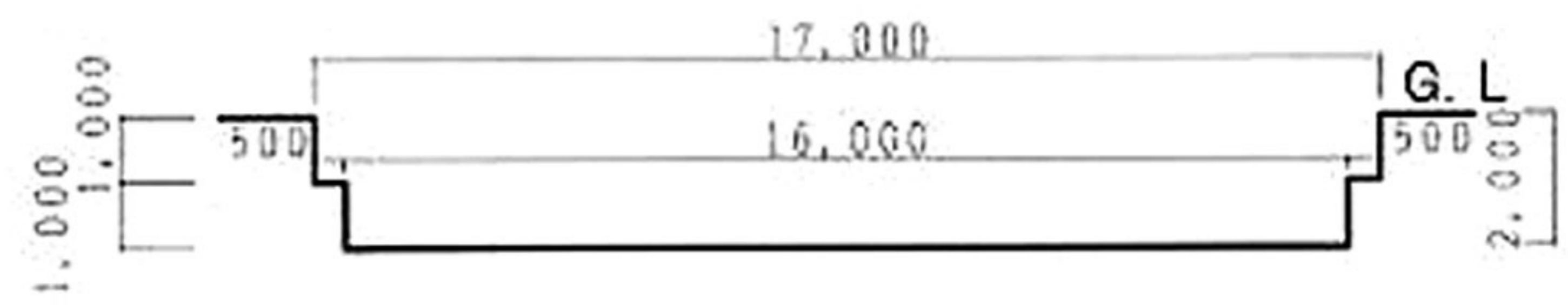
D-D' 断面図
