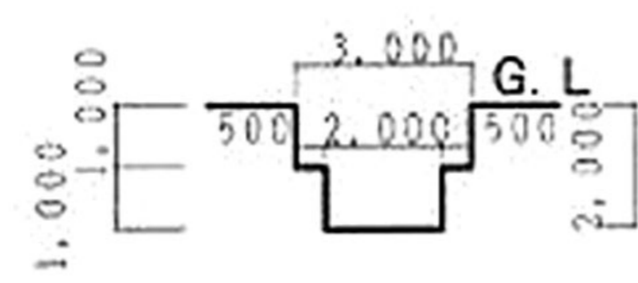
A-A' 断面図
