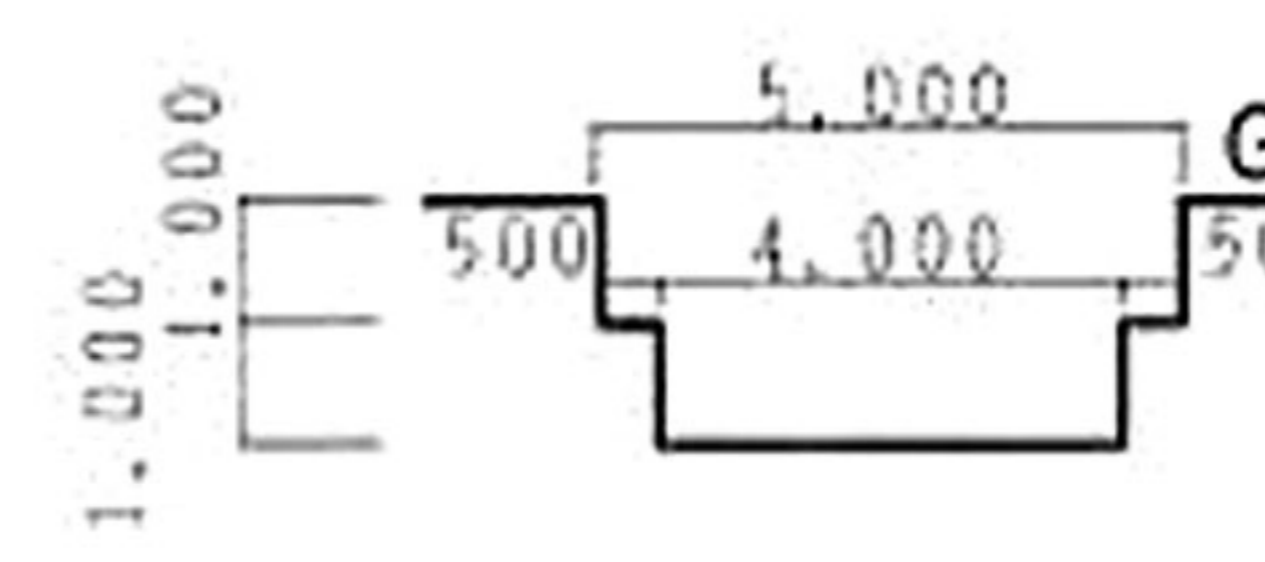
B-B' 断面図
