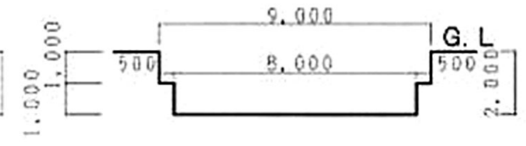
C-C' 断面図
